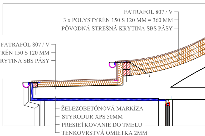
Detail 4 - napojenie strechy a markízy
