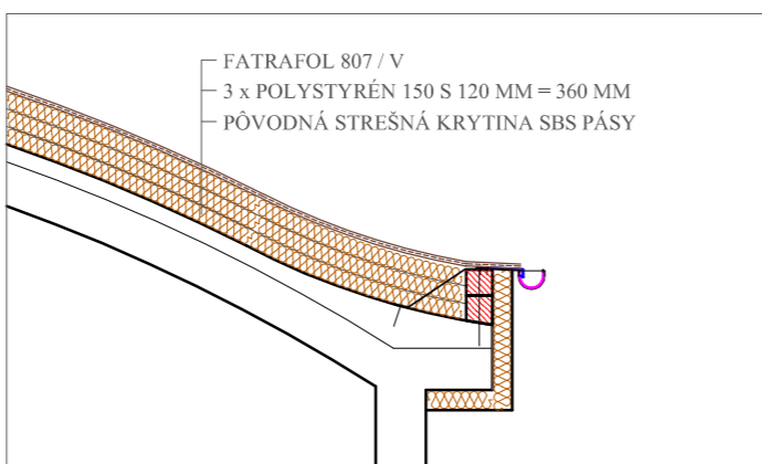
Detail 2 - vonkajší odkvap
