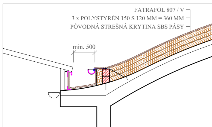
Detail 1 - vnútorný žľab striech
