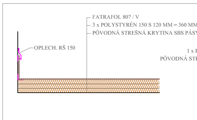
Detail 3 - napojenie na stenu
