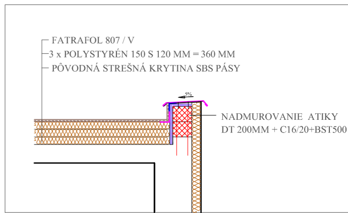
Detail 5 - ukončenie oblúkovej atiky
